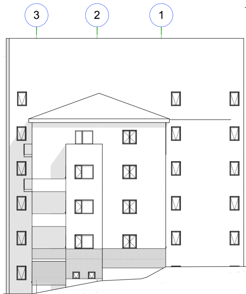
Øst Fasade 1:200
